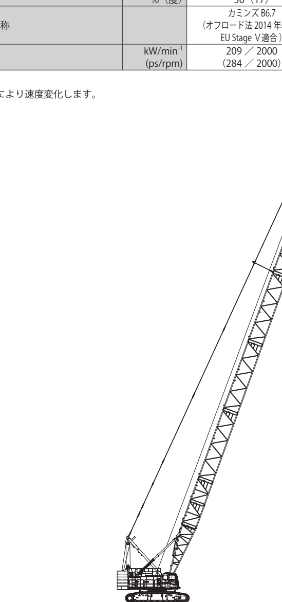
クレーン仕様ブーム最長
